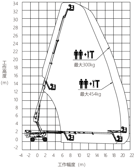
LT32JE性能曲线图
