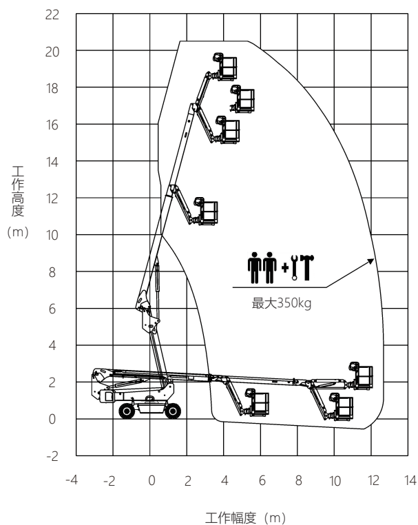
LT18JE-c 性能曲线图
