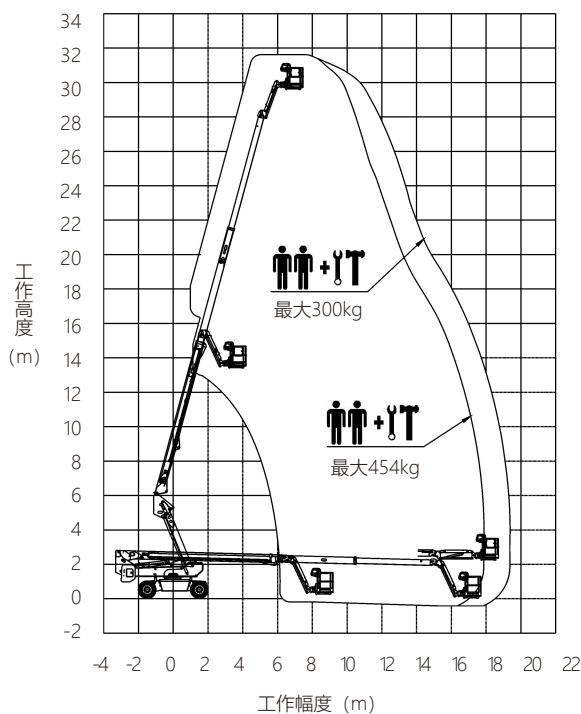
LT30JE-c 性能曲线图
