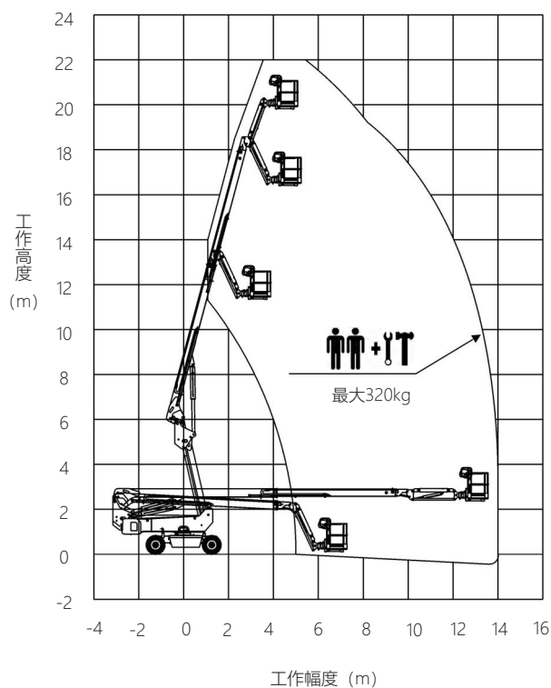
LT20JE-c 性能曲线图
