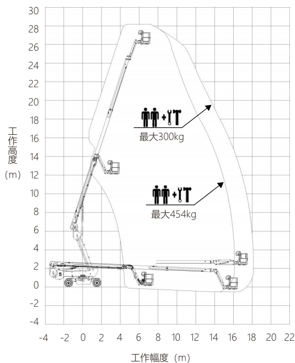
LT26JE-c 性能曲线图
