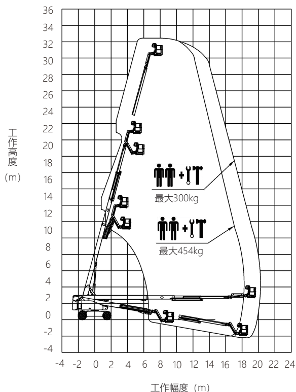
LT32JG4性能曲线图
